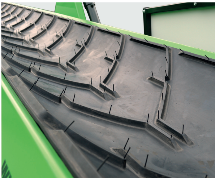
Transportband in trogvorm
